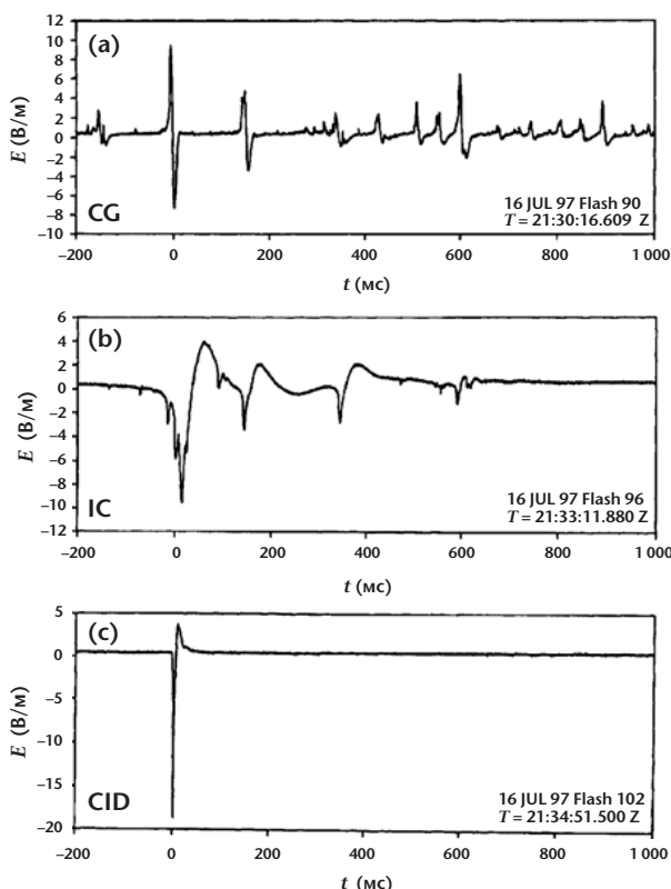
Рисунок 6.3. Примеры волновых форм импульсов электрического поля ( E ), характерных для (a) начального пробоя в отрицательных наземных вспышках по направлению от облака к земле (CG), (b) начального пробоя во вспышках внутри облака (IC) и (c) компактных внутриоблачных разрядов (CIDs). Положительно заряженное электрическое поле (правило знаков атмосферного электричества) отклоняется вверх. (Займствовано из работы Rakov, 1999).
