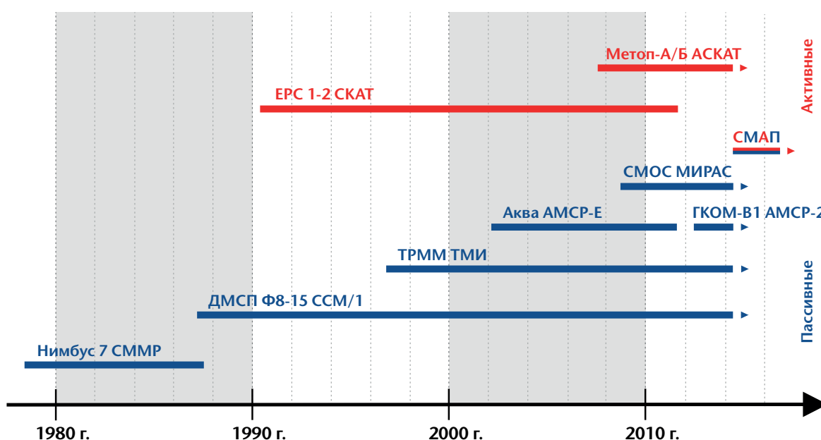
Рисунок 11.2. Активные и пассивные микроволновые датчики, используемые для получения данных о влажности почвы.
