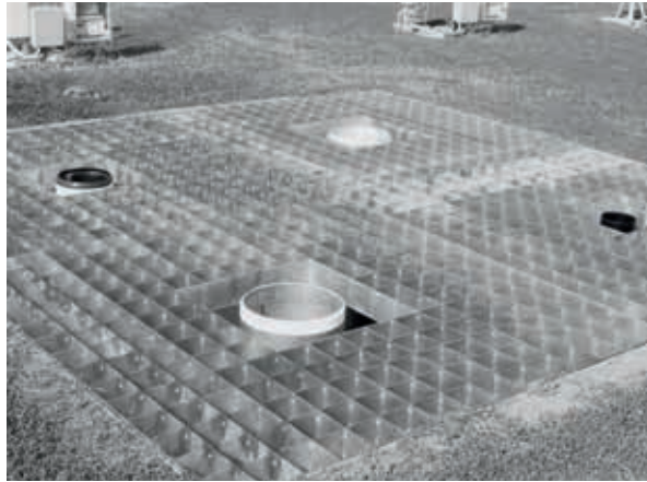
Рисунок 6.С.2. Установка эталонных осадкомеров ямочного типа на станции Винья-ди-Валле, Италия (2007 г.) во время проведения ВМО полевых взаимных сравнений измерений интенсивности осадков.
