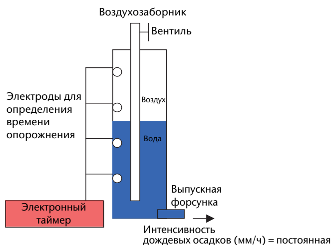
Упрощенная схема работы портативной полевой установки для калибровки.
